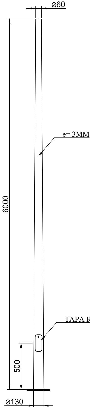
DETALLE POSTE s/e
