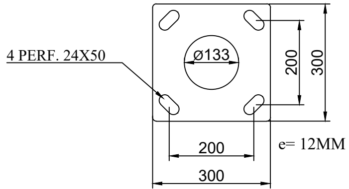
DETALLE PLACA BASE s/e
