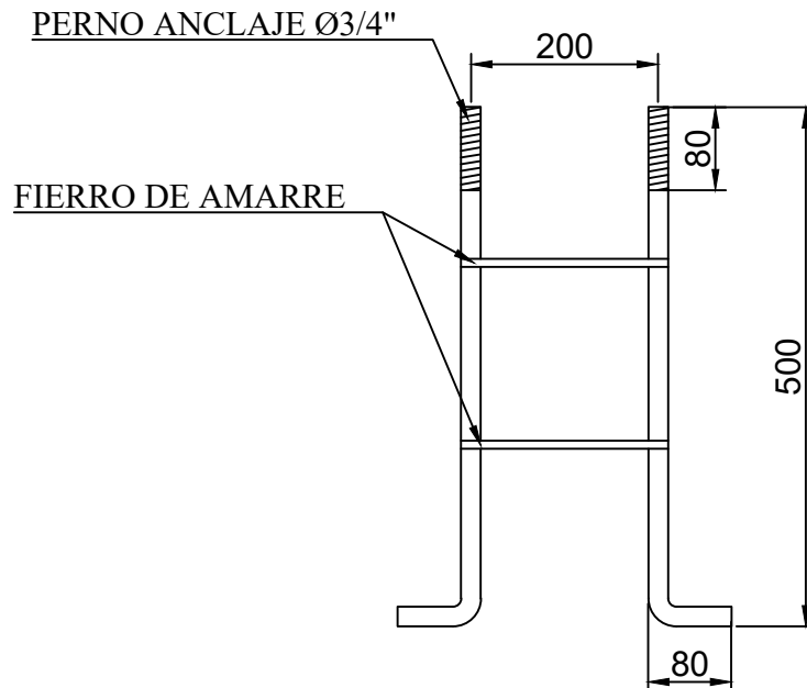
DETALLE CANASTILLO s/e
