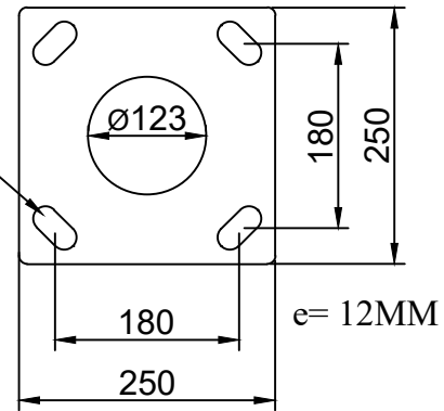
DETALLE PLACA BASE s/e
