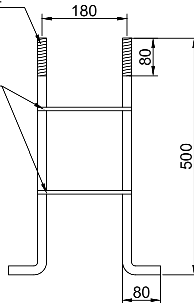
DETALLE CANASTILLO s/e
