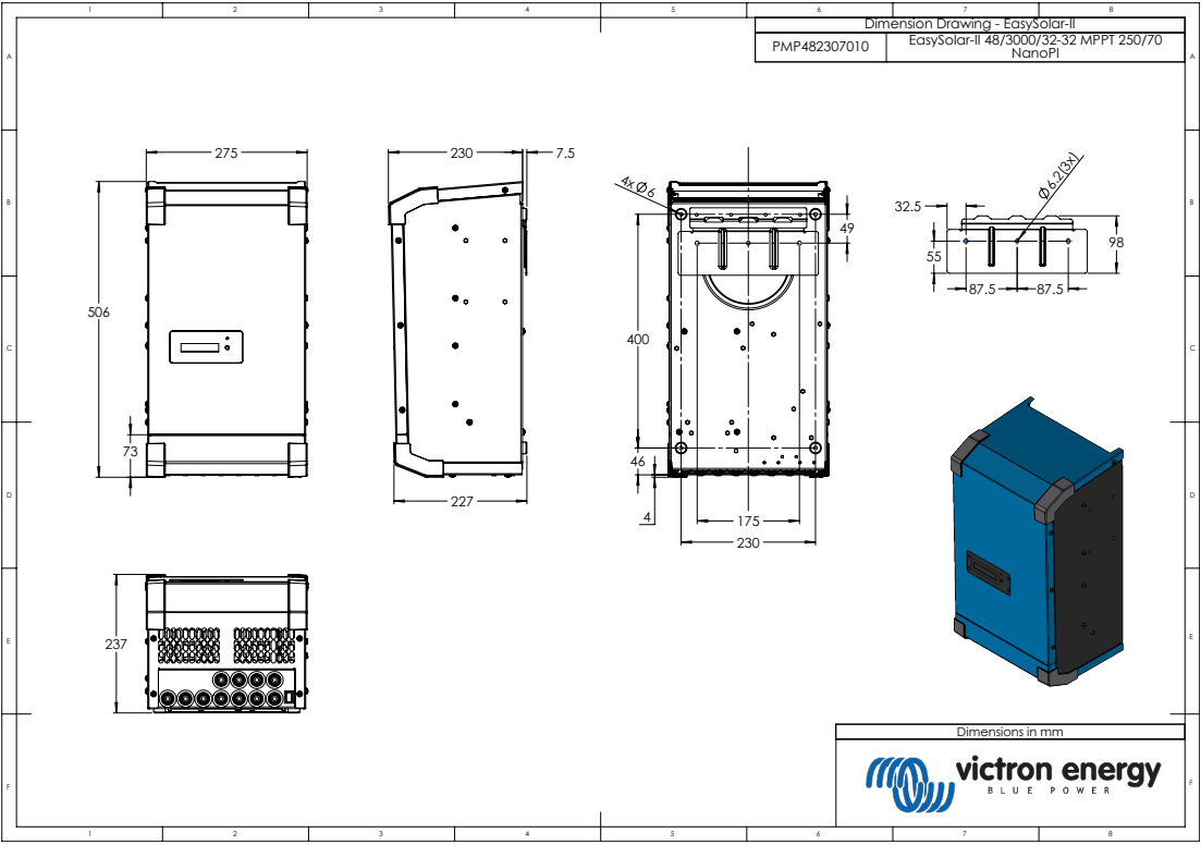
Esquema de dimensiones - EasySolar-II 48/3000/35-32 MPPT 250/70 GX - PMP482307010
