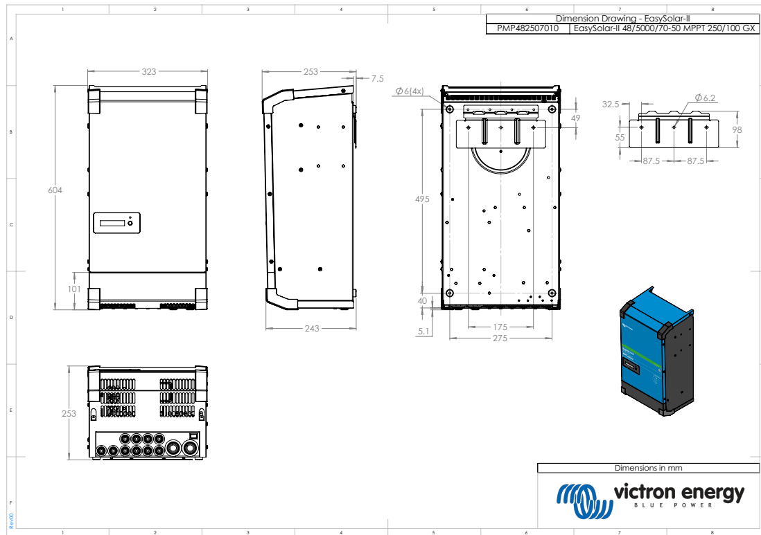
Esquema de dimensiones - EasySolar-II 48/5000/70-50 MPPT 250/100 GX - PMP482507010
