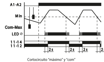
Cortocircuito "máximo" y "com"
