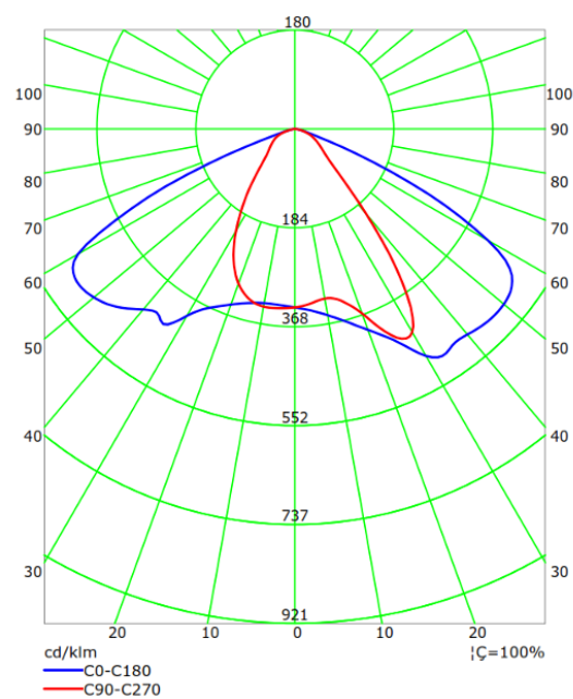
Curva de distribución de intensidad luminosa (cd/klm)
