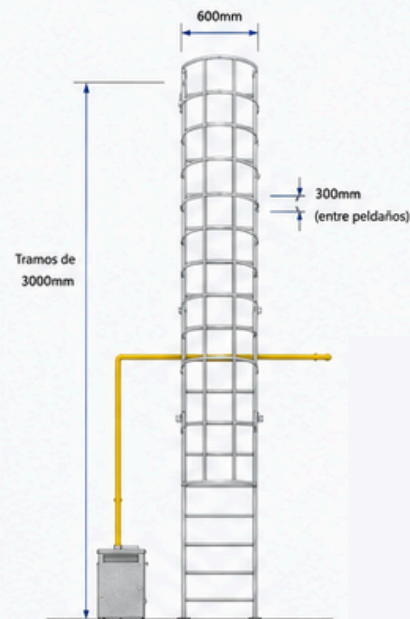
VISTA FRONTAL - ESCALERA COMPLETA
