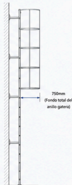
VISTA LATERAL - ESCALERA
