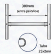
DETALLE PELDAÑO (TÍPICO)
