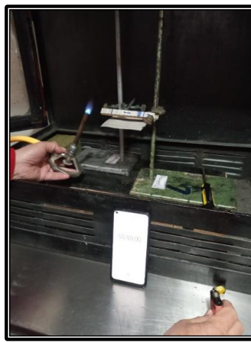
Figura 6.3 Probeta #1 durante el ensayo
