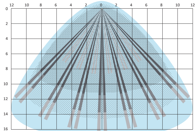
QDTP200H, QDTP200HM – Vista desde arriba
