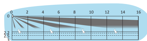
QDTP200H, QDTP200HM – Vista lateral
