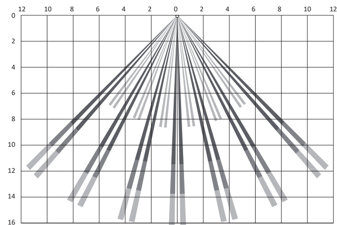
QIRP100H, QIRP200H – Vista desde arriba
