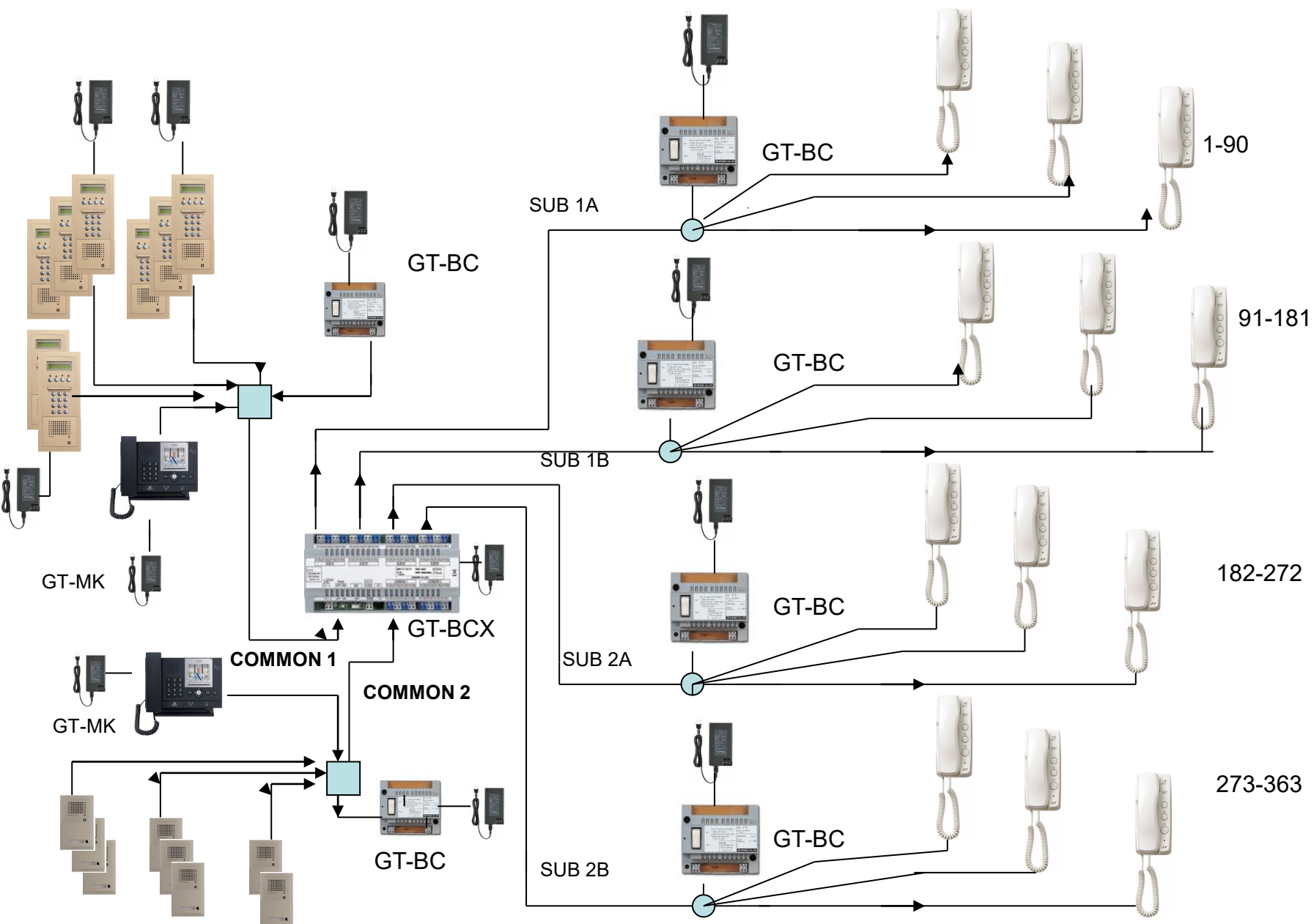
CONEXIÓN SIMPLIFICADA DE SISTEMA GT
