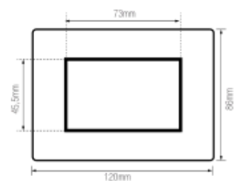
INTERRUPTOR TECLÓN 73mm
