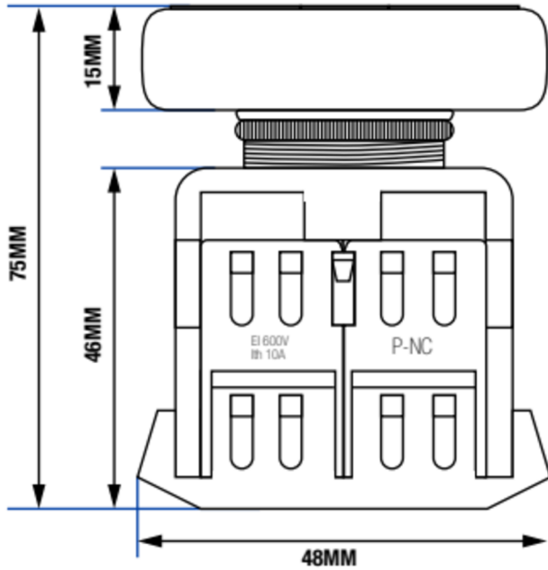
ESQUEMA 5370075
