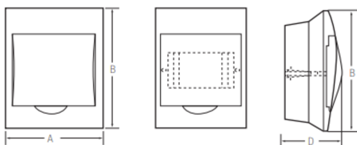
Dimensiones tapa
