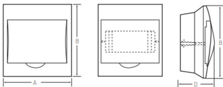
Dimensiones tapa
