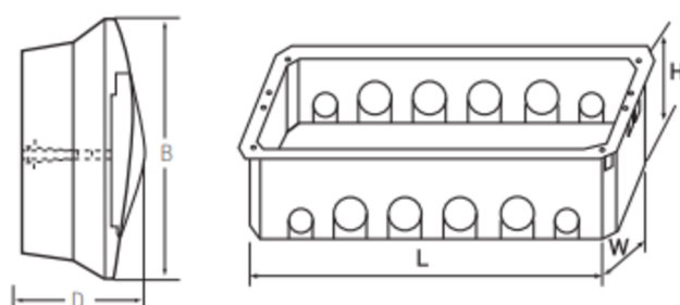
Dimensiones base
