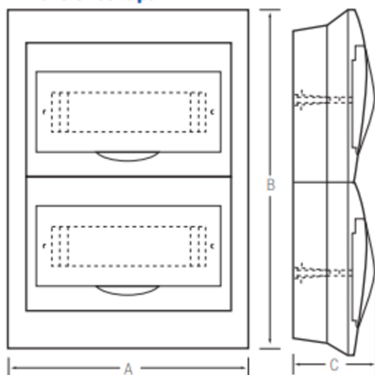
Dimensiones tapa
