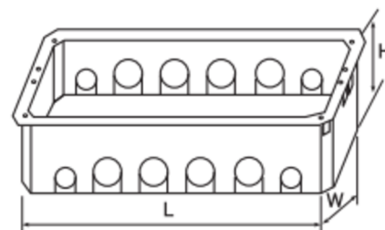
Dimensiones base
