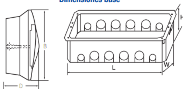
Dimensiones base
