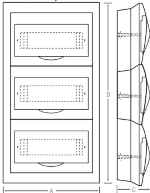
Dimensiones tapa
