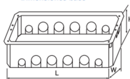
Dimensiones base
