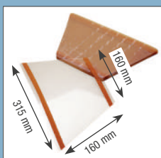
Resistencia calefactora
