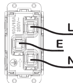
Esquema de conexión
