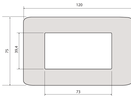
Placa tres puestos · mm
