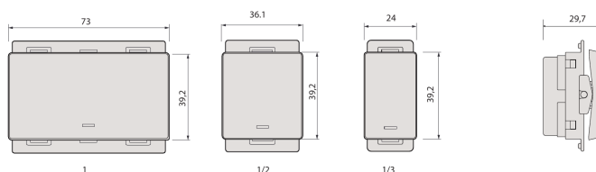
Módulos 1, 1/2 y 1/3 · vista lateral · medidas en mm
