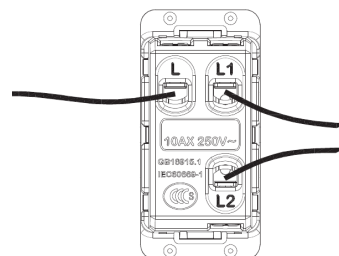
Esquema de conexión
